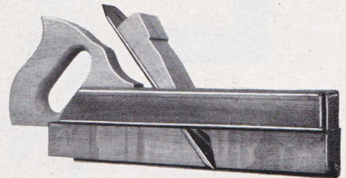
N° 47 BOUVET A JOINDRE 2 MORCEAUX LANGUETTE FER A POIGNÉE
